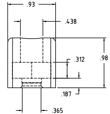
12449-SSNB Ⓐ
