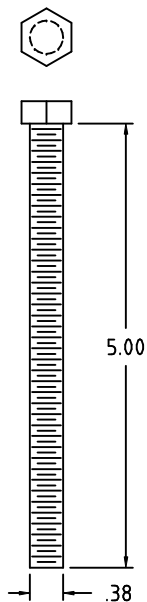
3/8-16X5" TYPE 304 SS BOLT 12463
